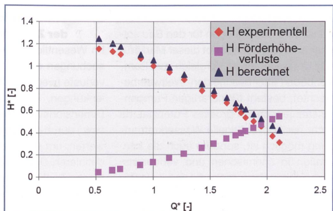
Bild 2. Modellierung der einen von fünf Testpumpen an der EIG mit berechneten und gemessenen Werte.
