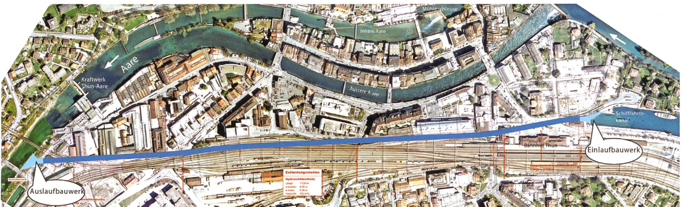
Bild 3. Entlastungstollen: Situation (Quelle: IC).
