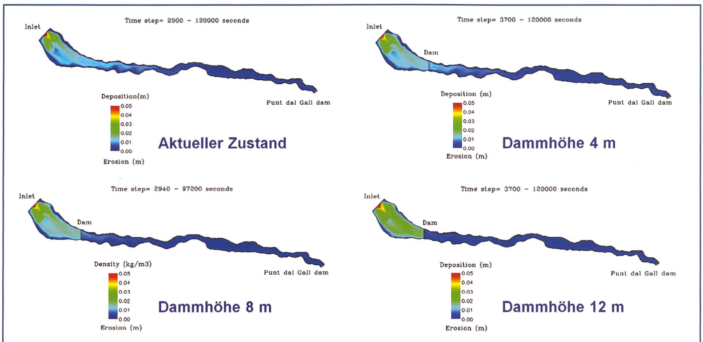
Bild 7. Ablagerungen am Seegrund für das Hochwasser 2000 mit einer Zuflussschwebstoffkonzentration von 15 g/l in Abhängigkeit der Schüttdammhöhe als Hindernis gegen Trübestrome.
