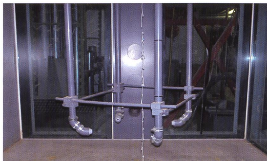
Bild 3. Versuchsanlage für kreisförmig angeordnete Düsen zur Erzeugung einer Aufwärtsströmung. Links: Detail einer Düse. Rechts: Düsenanordnung vor der Fassung Schemaskizze der mit dem Wasser der Beileitungen gespiesenen Wasserstrahlen in der Frontwand im Hintergrund (Jenzer et al. 2009).
