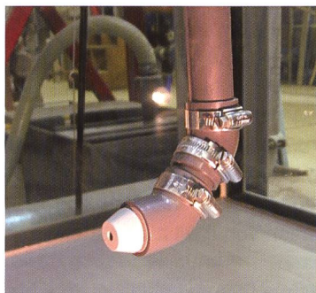
Bild 3. Versuchsanlage für kreisförmig angeordnete Düsen zur Erzeugung einer Aufwärtsströmung. Links: Detail einer Düse. Rechts: Düsenanordnung vor der Fassung Schemaskizze der mit dem Wasser der Beileitungen gespiesenen Wasserstrahlen in der Frontwand im Hintergrund (Jenzer et al. 2009).
