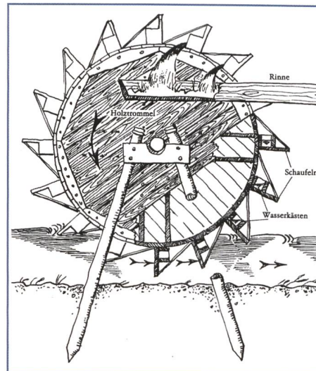
Bild 3.1. Schöpfrad nach Vitruv.
