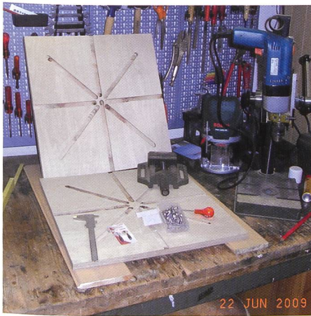
Bild 5.1. Beile Seitenwände des unterläufigen Wasserrads.
