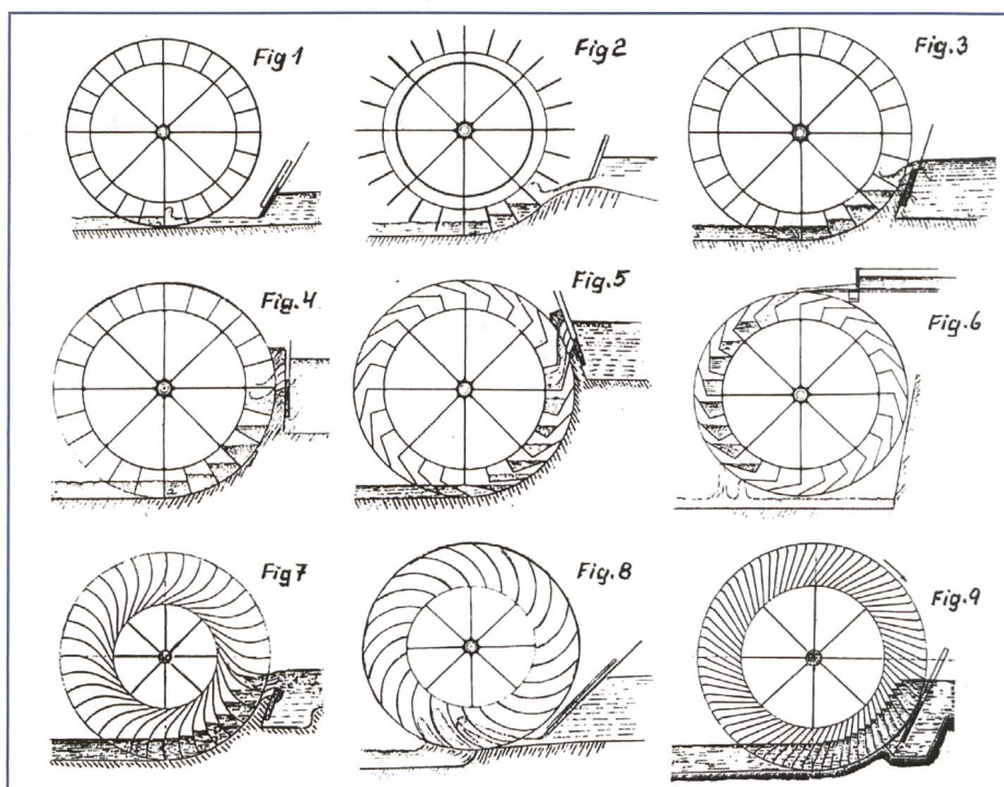
Bild 3.4. Wasserradtypen.
