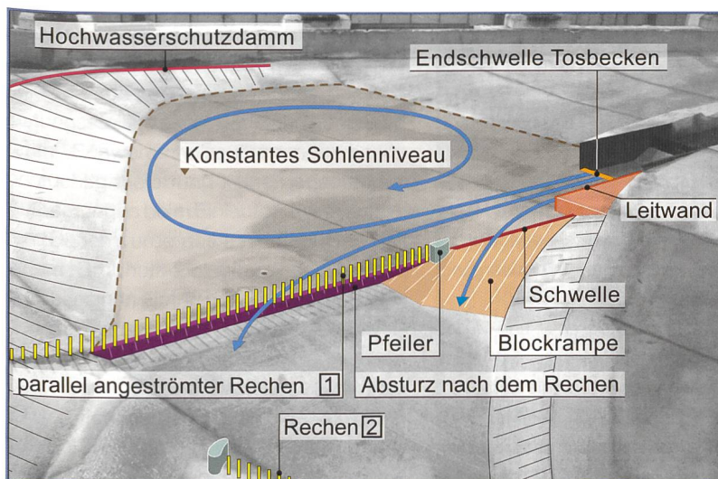
Bild 10. Links: Darstellung des optimierten Holzurückhalterums mit parallel angeströmtem Rechen (Blick gegen die Strömungsrichtung). Rechts: Detail des optimierten Unterwasserbereichs mit einem zweiten Rechen.
