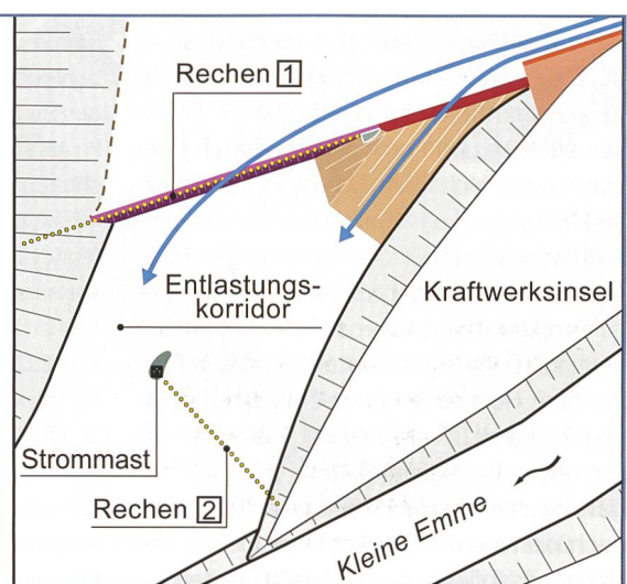
Bild 10. Links: Darstellung des optimierten Holzurückhalterums mit parallel angeströmtem Rechen (Blick gegen die Strömungsrichtung). Rechts: Detail des optimierten Unterwasserbereichs mit einem zweiten Rechen.
