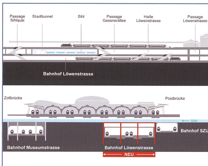
Bild 3. Querschnitt der Sihl im Bereich des Zürcher Hauptbahnhofes mit Oberbahnhof, Sihl und neuem Bahnhof Löwenstrasse (oben). Längsschnitt der Sihl im Bereich des Zürcher Hauptbahnhofes mit Oberbahnhof, Sihl und neuem Bahnhof Löwenstrasse (rot) neben den bestehenden unterirdischen Bahnhöfen Museumstrasse und SZU (unten) (Quelle: SBB).
