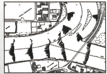
Strömungsvektoren
