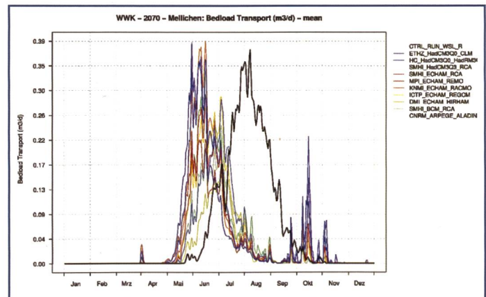
Bild 8. Jährliche Geschiebeganglinien ( \text{m}^3/\text{Tag} ) für je zehn Szenarien der Perioden 2021 bis 2050 (links) und 2070 bis 2099 (rechts), jeweils im Vergleich zur Referenzperiode 1980–2009 (schwarz) für das Einzugsgebiet Mellichen (Grande Dixence).
