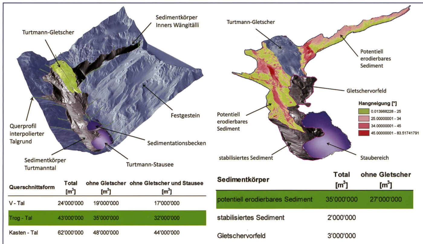
Bild 9a. Die Sedimentkörper im oberen Turtmanntal und im Innern Wängitäl.
