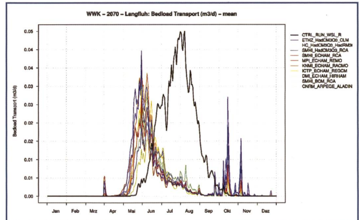
Bild 7. Jährliche Geschiebeganglinien ( \text{m}^3/\text{Tag} ) für je zehn Szenarien der Perioden 2021 bis 2050 (links) und 2070 bis 2099 (rechts) im Vergleich zur Referenzperiode 1980–2009 (schwarz) für das Einzugsgebiet Langfluh (Grande Dixence). Klar erkennbar ist die saisonale Verschiebung der Geschiebelieferung von den Sommermonaten (glazial) zum Frühling (nival).
