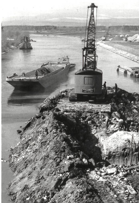
Bild 7. Aushub der letzten Verengung bei Sugiez im Broyekanal während der Zweiten Juragewässerkorrektur. (archiv suzanne muller).
