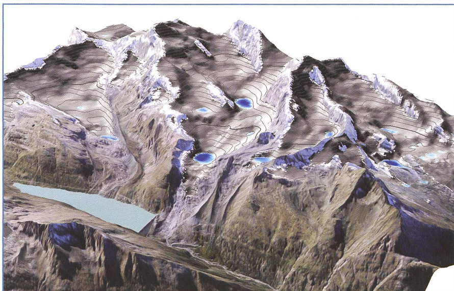
Bild 11. Die modellierten Gletscherbetten der Region Mattmark. In der Bildmitte das Bett des Allalingsgletschers mit zwei grösseren modellierten Übertiefungen (potenzielle Seen). Reproduziert mit Bewilligung von swisstopo (BA110005).
