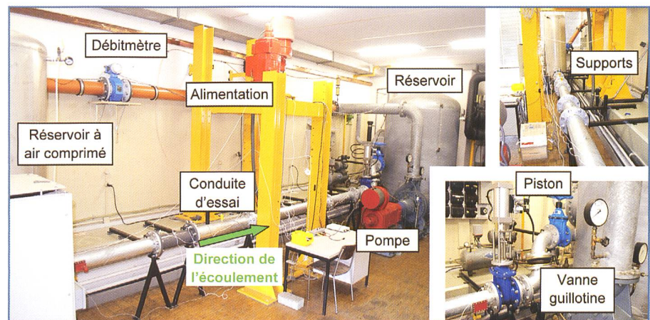
Figure 4. Modèle physique à échelle réduite construit au Laboratoire de Machines Hydrauliques (LMH) de l'Ecole Polytechnique Fédérale de Lausanne (EPFL).
