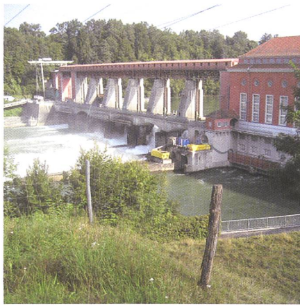
Bild 2. KW Eglisau-Glattfelden (Foto: SWV/Pfa).
