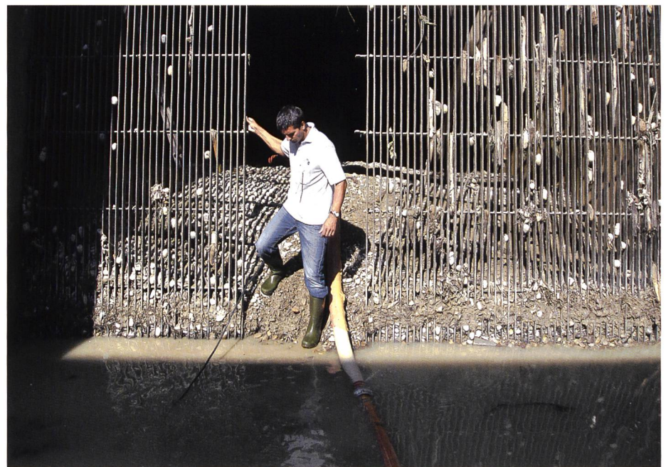
Bild 8. Vorgefundene Ablagerungen hinter dem Rechen, nachdem die Stauhaltung Ende September 2011 aufgegeben und die gesamte Wasserfassung sowie die Turbineneinläufe entwässert worden waren.
