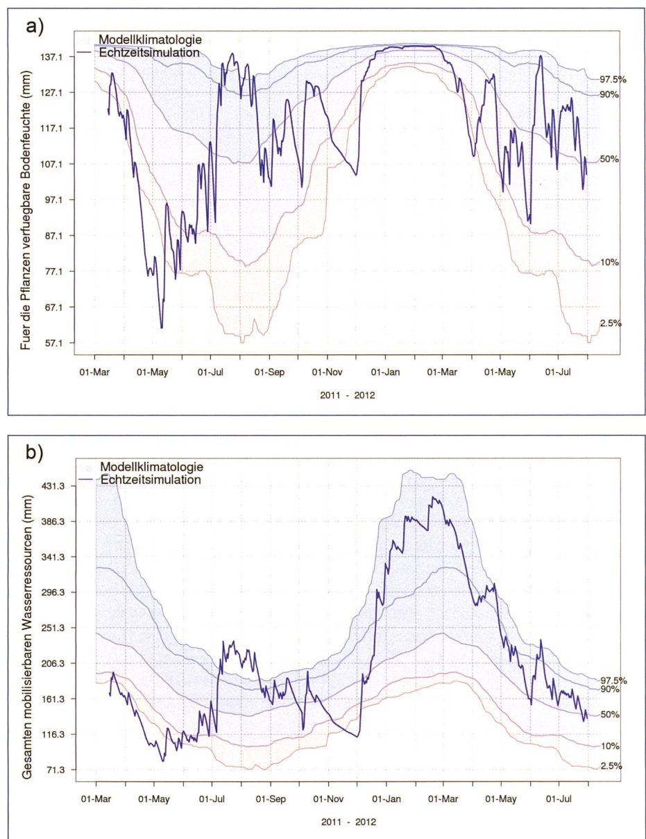
Bild 3. Modellerte Klimatologie (Zeitraum: 1980–2009; farbige Flächen im Hintergrund) und operationelle Simulation respektive Vorhersage (ausgezogene Linie) der Bodenfeuchte (a) sowie der gesamten mobilisierbaren Wasserressourcen (b) im Einzugsgebiet der Thur für den Zeitraum März 2011 bis Juli 2012.
