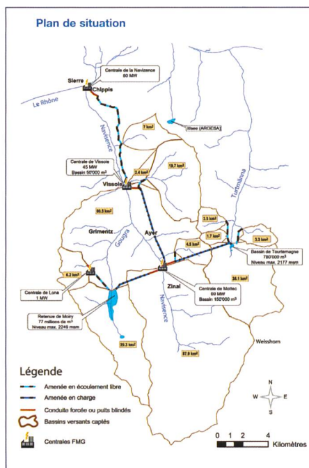
Bild 3. Einzugsgebiet der Kraftwerke Gougria SA mit der Zentrale Navisence in Chippis bei Sierre (Quelle: FM Gougria).
