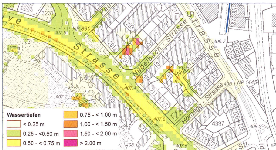
Bild 2. Überlagerte Maximalwerte der Wassertiefen aus 2D-hydronumerischen Modellierungsergebnissen des Hornbaches bei HQ 100 .
