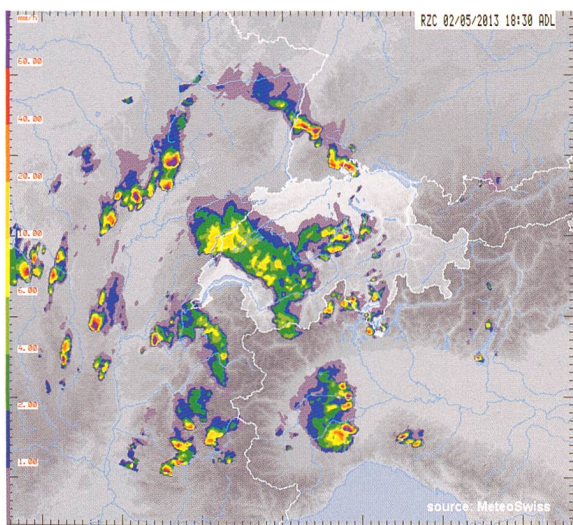
Bild 6. Am 2. Mai wütete über Schaffhausen SH ein Gewitter mit Rekordniederschlägen (Grafik: MeteoSchweiz). In Schleithem SH führte das Donaubächli Hochwasser (Foto: Peter Fürst).
