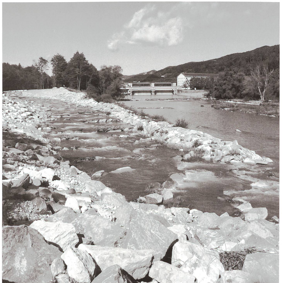
Bild 20. Umgehungsgewässer beim Kraftwerk Ruppertswil-Auenstein.
