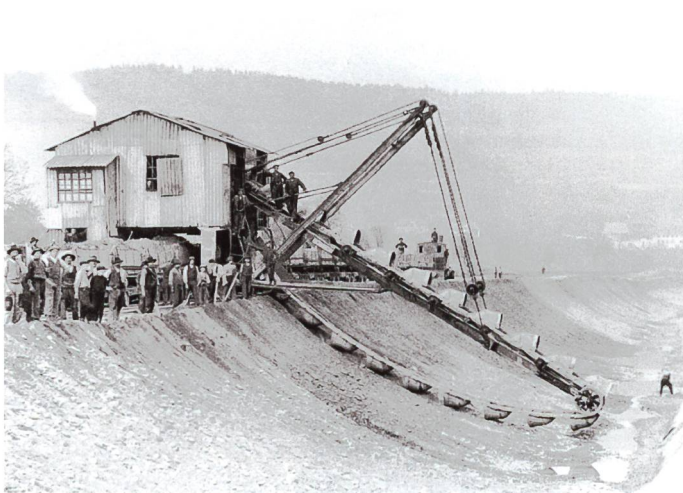
Bild 4. Der dampfbetriebene Kettenbagger bei den Aushubarbeiten für den Kanal beim Kraftwerk Aarau Anno 1910.
