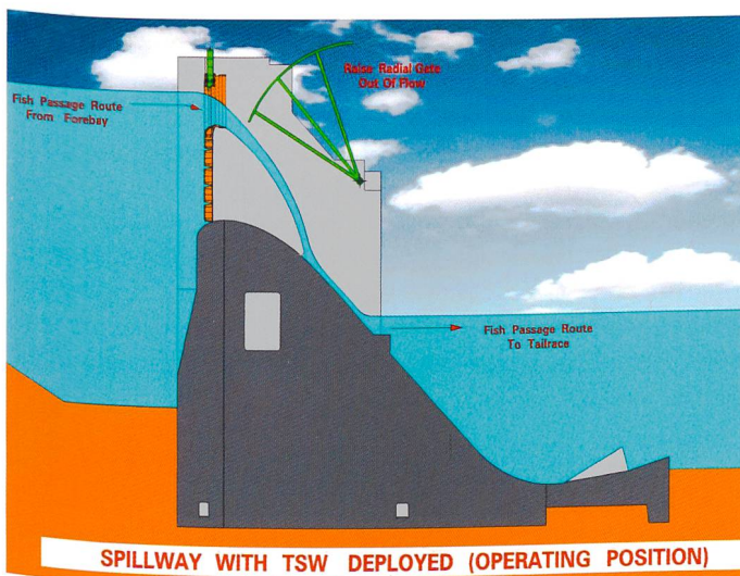
Bild 12. Temporärer Wehrrücklaufkörper zur oberflächennahen Wehrpassage (Temporary Spillway Weir) (Quelle: Hockersmith 2013).
