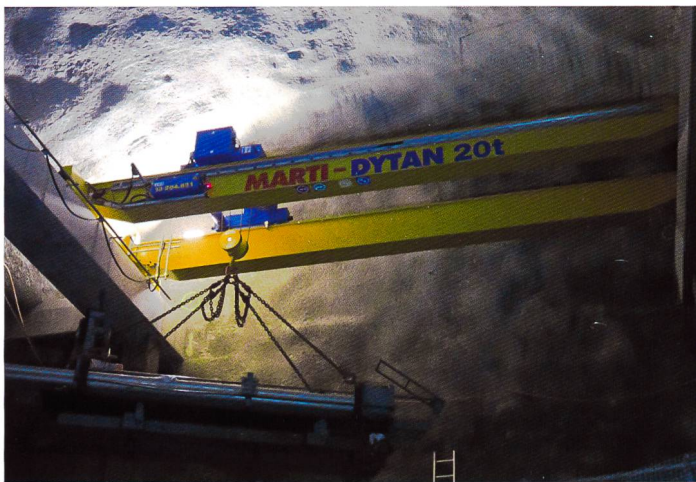
Bild 1. Der 20 t Zweiträger-Laufkran bringt die neuen Druckrohre in den Stollen ein.
