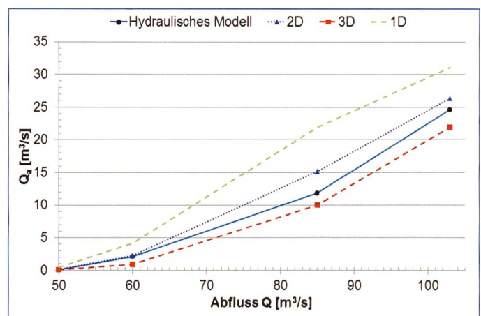
Bild 7. Ausleitcharakteristika.
