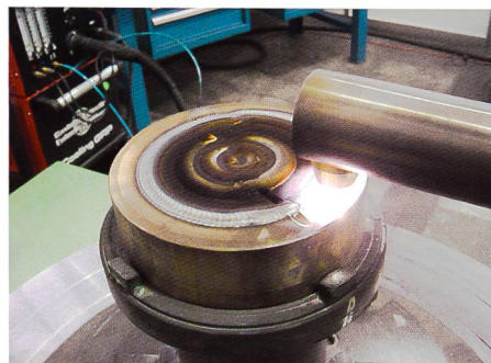
Bild 3. Versuchsplatte mit PTA geschweisst.
