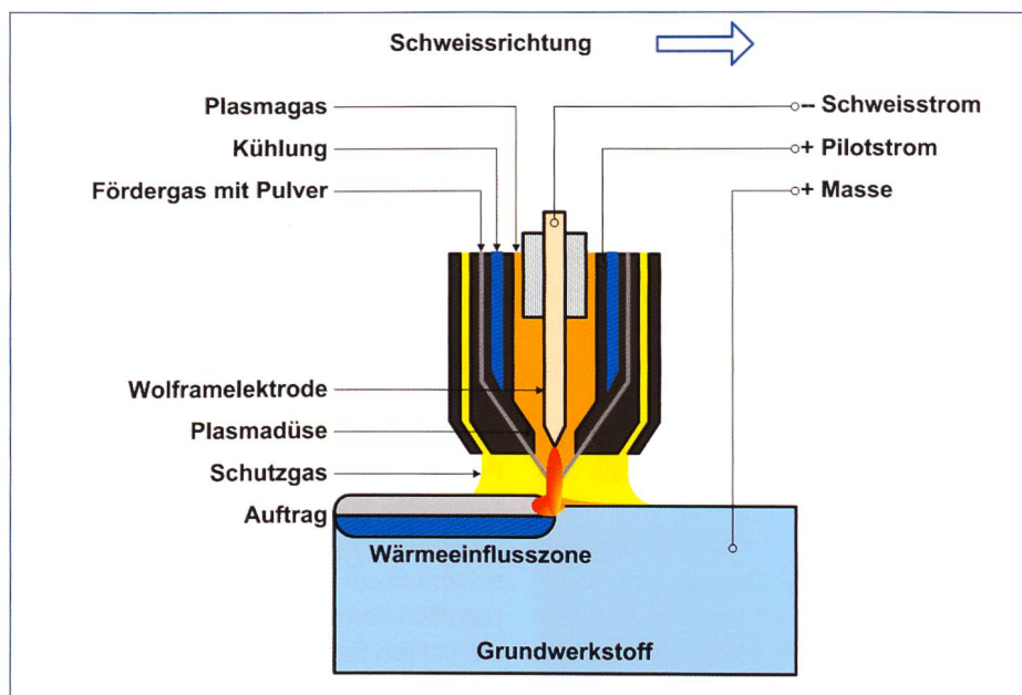
Bild 1. Verfahrensprinzip PTA-Auftragschweißen.
