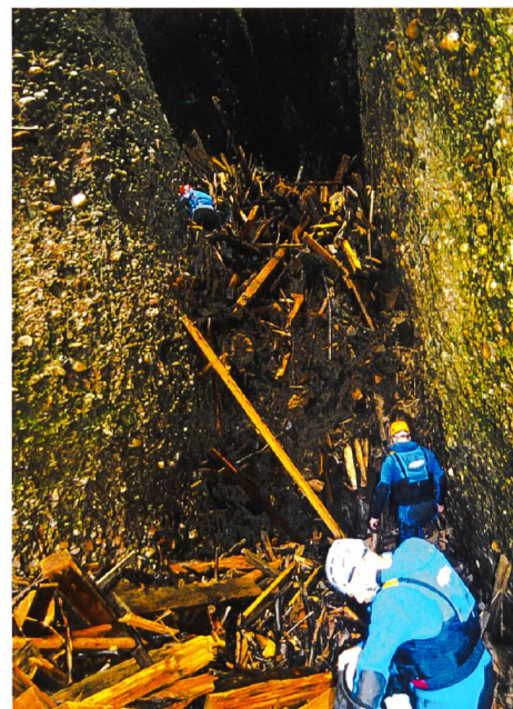
Bild 2. Links: Begehung der Verklauung der Brücke über den Sädelgrabe (Foto: Geotest AG); rechts: Verklauung im Räbloch (Foto: Feuerwehr Eggwil).
