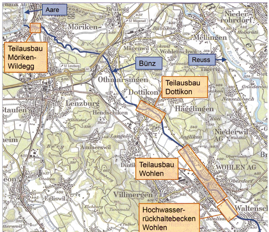
Bild 1. Teilprojekte des Regionalen Hochwasserschutzes Bünztal.
