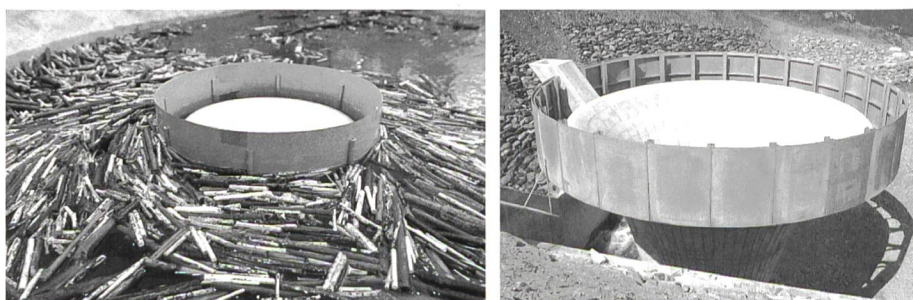
Bild 6. Tulpe mit Tauchwand im Geschiebesammler am Kelchbach in Naters, Kanton Wallis; Durchmesser der Tulpe ca. 14 m. Links: Modellversuch; rechts: Prototyp (Fotos: Lange und Bezzola, 2006).
