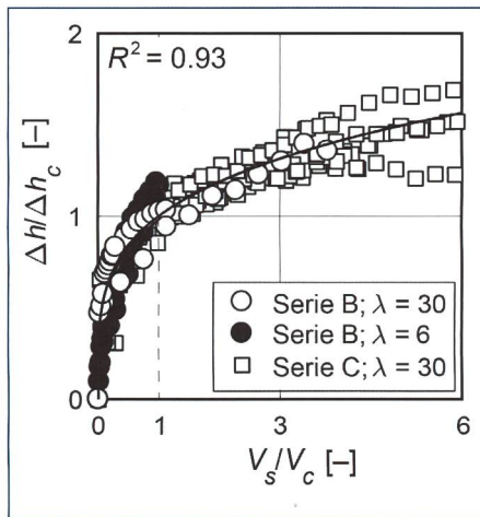
Bild 9. Aufstauverhältnis \eta = \Delta h / \Delta h_c versus relatives Schwemmholzvolumen V_s / V_c mit Gl. (6).
