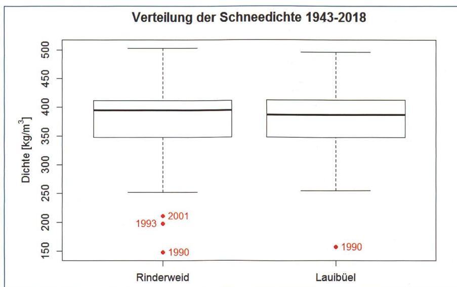
Bild 9. Box-Plot-Darstellung der ermittelten Schneedichten für die Messorte Rinderweid und Lauibüel über die Messreihe 1943–2018 (jeweils am 1. April).
