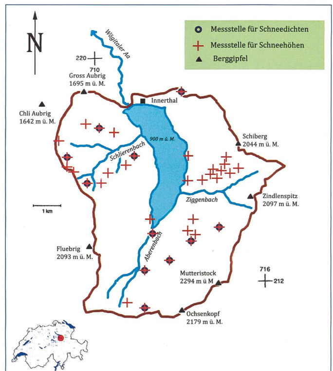
Bild 3, rechts. Einzugsgebiet des Wägitalersees mit dem eingezeichneten Schneemessnetz.
