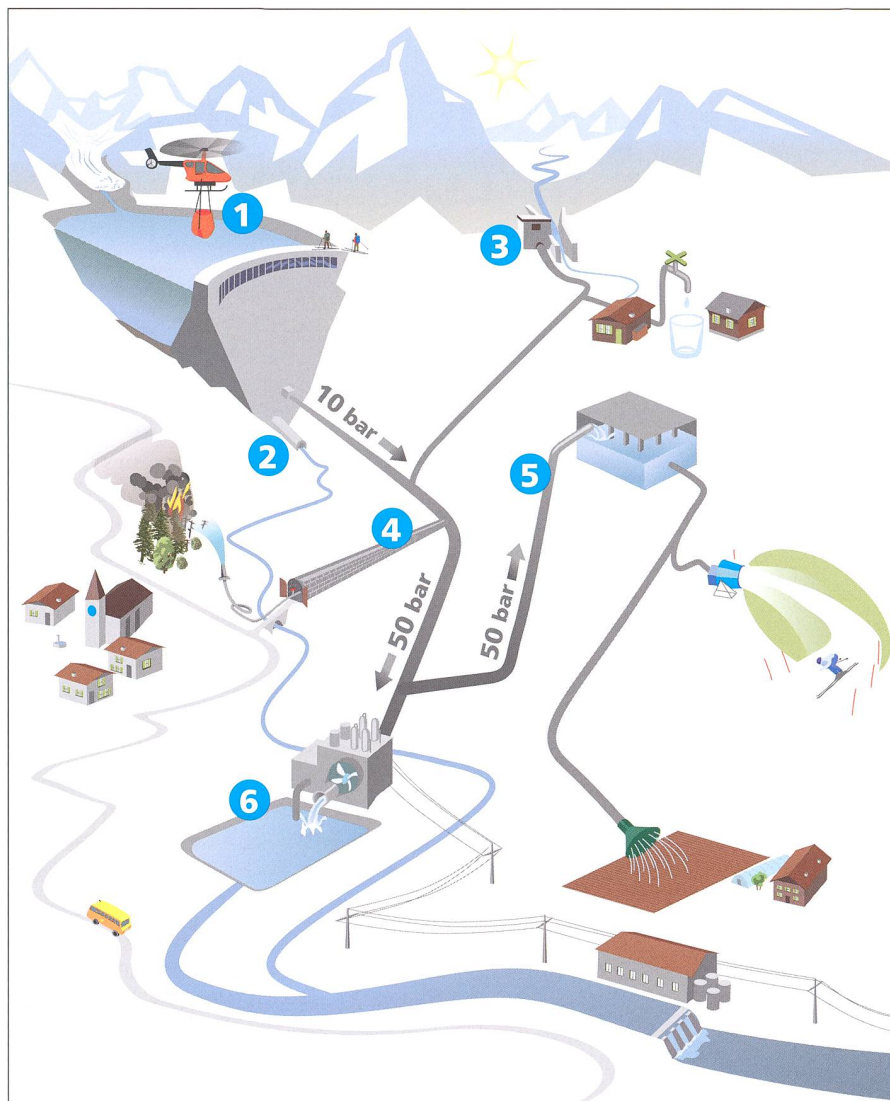
Bild 1: Darstellung der potenziellen Wasserentnahmestellen aus einem Speicherkraftwerksystem (Quelle: Valentin Rüegg in Zusammenarbeit mit Philippe Roth und Astrid Björnsen Gurung).
