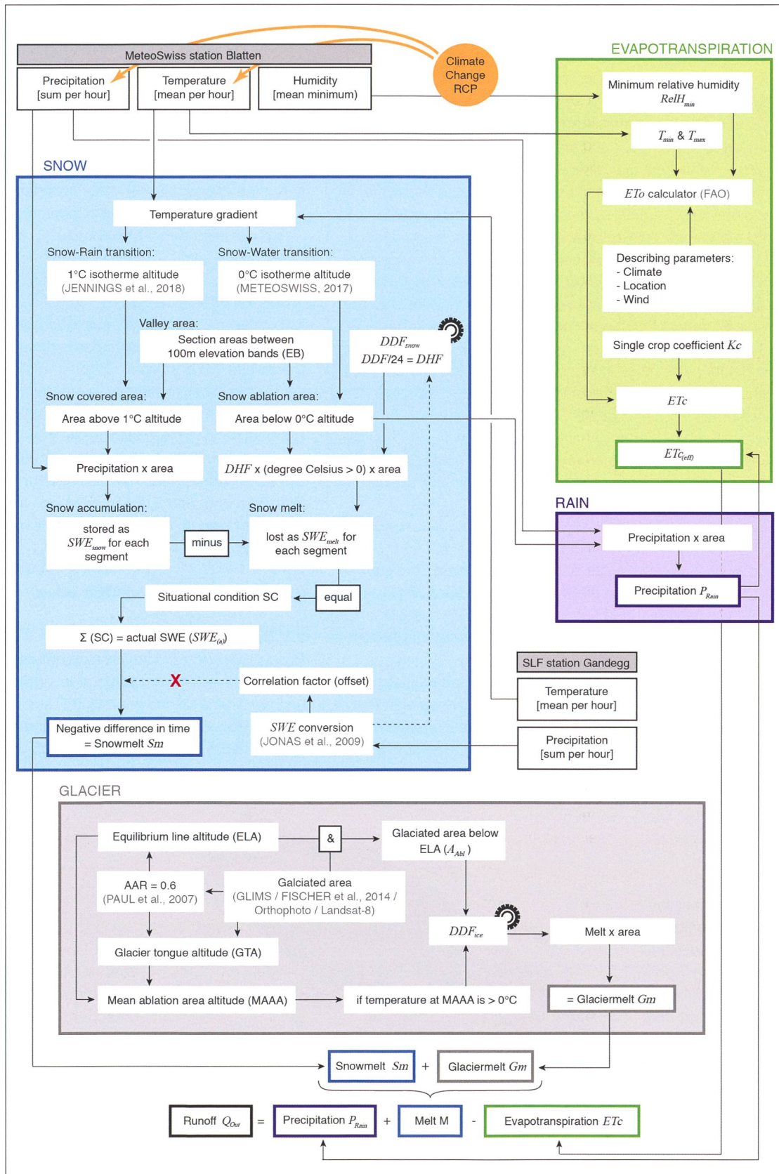
Bild 2: Das verwendete hydrologische Modell. Ausgehend von den Messwerten der Meteostation Blatten und Daten der Gletscherfläche, wurden alle Parameter zur Abflussbestimmung berechnet. Die Faktoren, welche mit einem Zahnrad versehen sind, dienen zur Kalibrierung des Modells.
