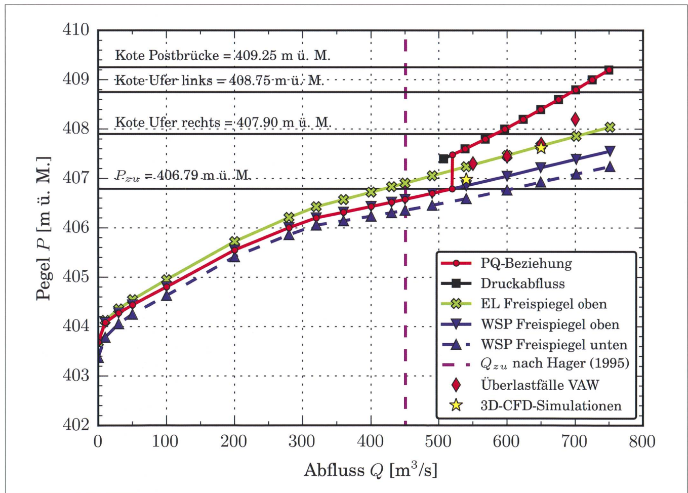
Bild 9: PQ-Beziehung des Sihldurchlasses unter Berücksichtigung von Druckabfluss (Kapitel 4.3) für das Szenario mit 0,4 m Auflandung, ohne Verkläuerung und Einhaltung der Unterhardbedingung (Abfluss Sihl und Limmat zusammen maximal 600 \text{ m}^3/\text{s} ). Als Anhaltspunkte sind die Überlastfälle der VAW, 3D-CFD-Simulationen und Q_{zu} gemäss Ansatz nach Hager (Gleichung 7) dargestellt. Die Energielinie (EL) und der Wasserspiegel (WSP) oben/unten für den Freispiegelabfluss stammen aus dem lokalen 2D-Modell.
