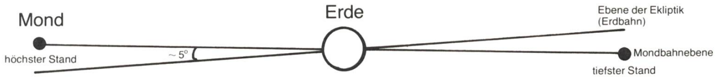
Abbildung 5: Schiefe der Mondbahn (Ansicht von der Seite). Der Abstand des Mondes von der Erde ist in der Skizze nicht im richtigen Massstab gezeichnet. Er müsste, richtig gezeichnet, viermal verlängert werden.
