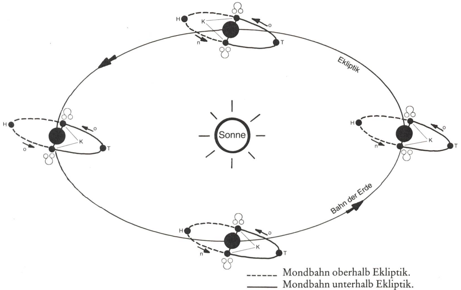
Abbildung 6: Die Bahnen der Erde und des Mondes zur Erklärung von obsigänt und nidsigänt. o: obsigänt, n: nidsigänt, K: Knotenlinie, T: tiefster Stand des Mondes, H: höchster Stand des Mondes, \circ\circ : aufsteigender Mondknoten, \infty\infty : absteigender Mondknoten.
