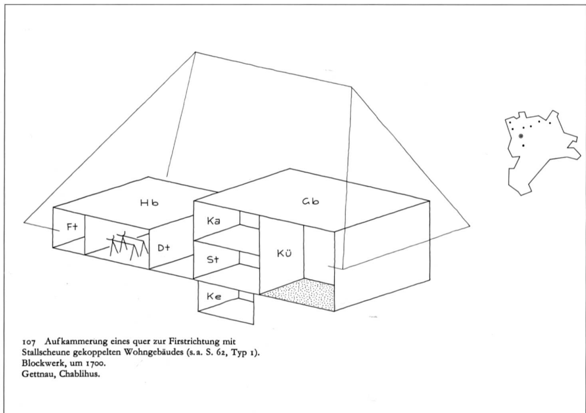
Aufkammerung des quer zur Firstrichtung mit Stallscheune gekoppelten Wohngebäudes, Gettnau, Chablihus. Ft: Futtertenne, Hb: Heubühne, Dt: Dreschtenne, Gb: Garbenbühne, Ka: Kammer, St: Stube, Ke: Keller, Kü: Küche. Quelle Ernst Brunner
