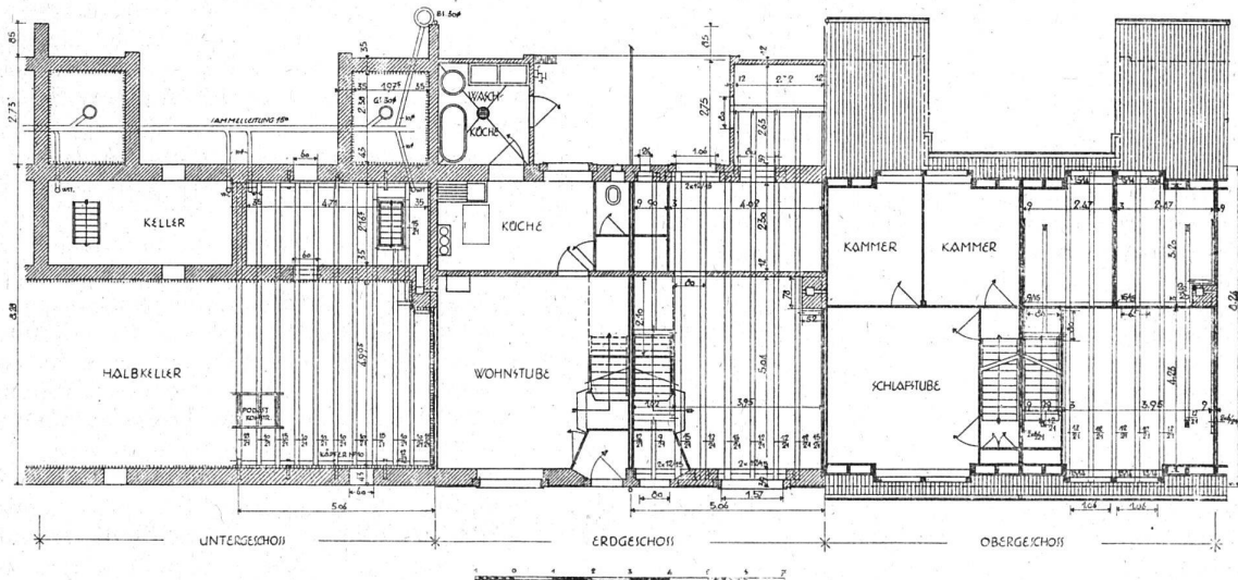
Grundrisse — Plans.
