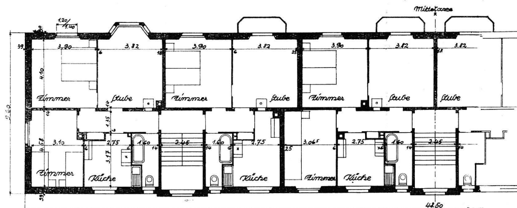
Grundriss Block II E (Rölfe).
