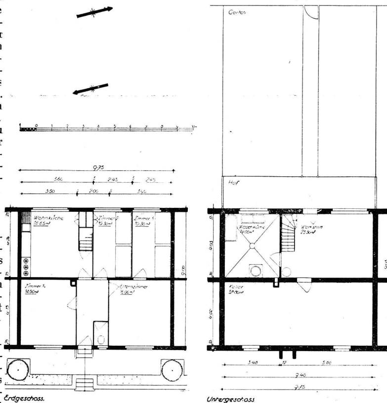
Grundriss des Projektes der Wohngenosenschaft „Lange Erlen“, Basel.
