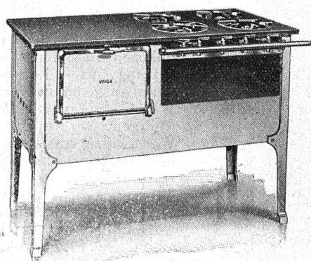
Fig. 2. Gasherd mit halbhochliegendem Bratofen und warmer Abstellplatte über dem letzteren.
