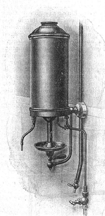
Fig. 5. Gasbetriebener Kleinwarmwassererhitzer für Küchen, Toiletten, Coiffeurgeschäfte etc.
