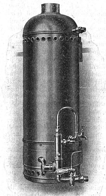
Fig. 9. Gas-Heißwasser-Stromautomat (ausgebaut mit Kupferrohrschlangen) für zentrale Warmwasserversorgung.
