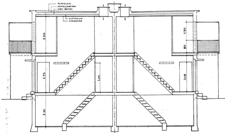
Kreuzreihenhäuser Schnitt
