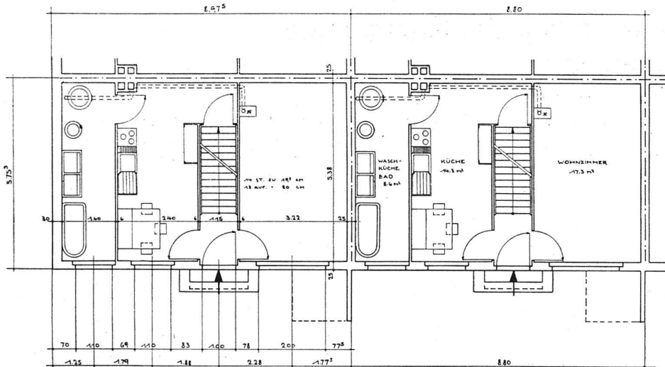
Kreuzreihenhäuser Obergeschoss
