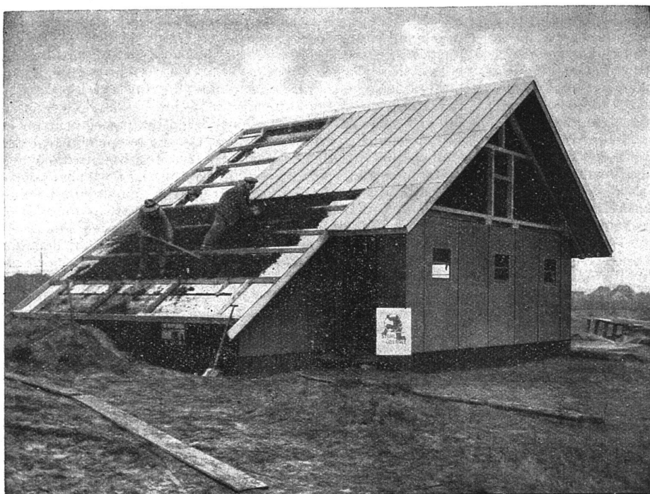
Stahllamellen-Siedlungshaus im Bau
