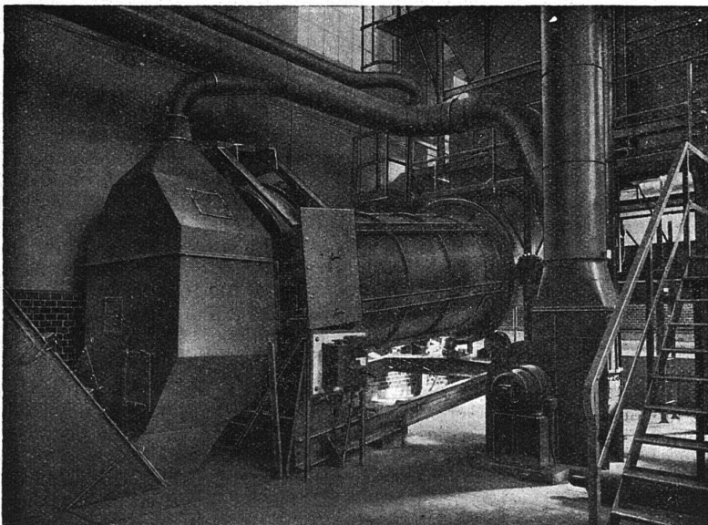
Müll-Sieb und Mischtrommel mit Magnetabscheider
