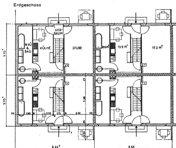
Erdgeschoss
