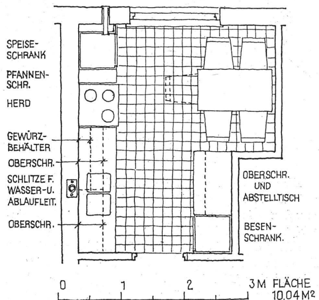
Abb. 2 b. Grundriß der schwedischen Standardküche
