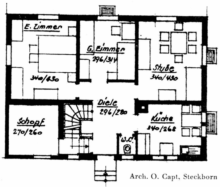
Erdgeschoß
