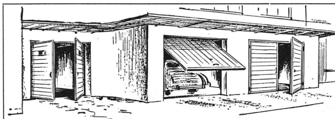
Schwenktore
