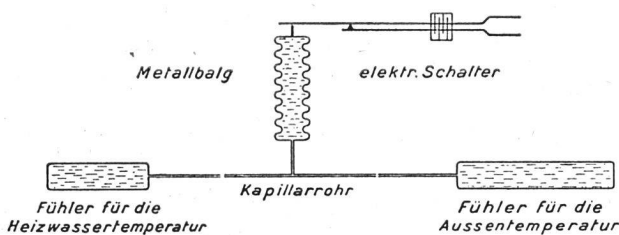
Schematische Darstellung einer Außensteuerung nach dem thermostatischen Prinzip
