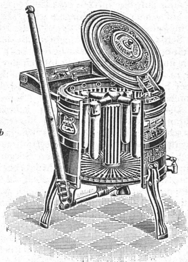
Bottichwaschmaschine mit Pendelunterantrieb
