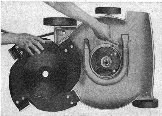
Dank dem wirkungsvollen Auspufftopf und der auf niedriger Tourenzahl drehenden 4-Messer-Scheibe ist der Rapid-Rasenmäher leiser.
