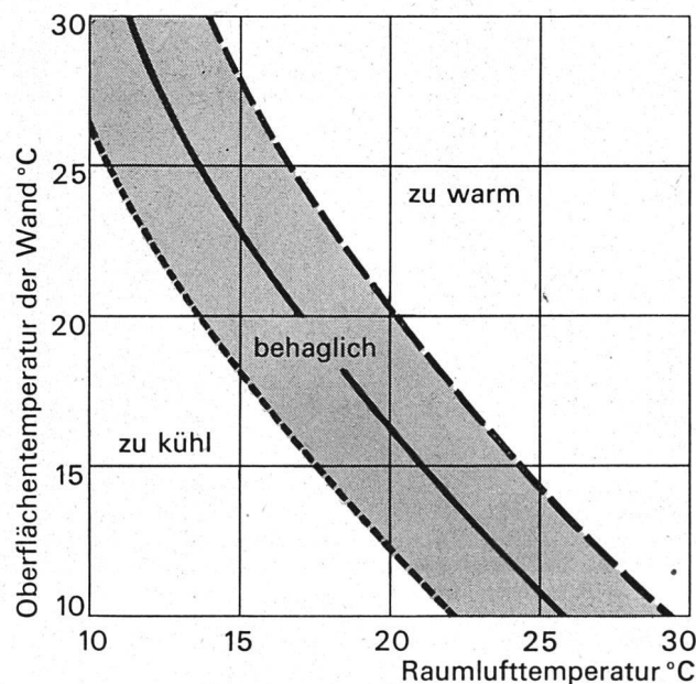
Behaglichkeitsempfindungen bei verschiedenen Wand- und Lufttemperaturen beheizter Räume
