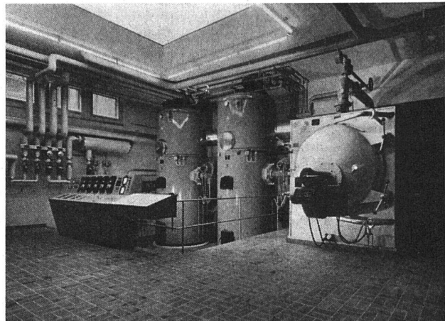
Heizzentrale der Baugenossenschaft Rotach in Zürich 3. Angeschlossen sind 31 Häuser mit insgesamt 306 Wohnungen und 7 Ladenlokalen. 1 Kessel zu 1 600 000 kcal/h, 2 Kessel à 500 000 mit 2 Boilern à 2000 Liter für die zentrale Warmwasserversorgung
