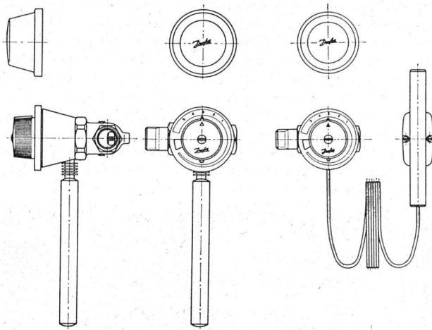
Thermostatische Heizkörperventile mit festem Fühler mit loseem Fühler
