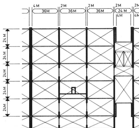
Primärstruktur
