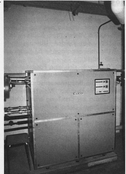
◀ Speicher und Kompressor der neuen Wärmepumpenanlage der Baugenossenschaft «Züri Leu» in Regensdorf. ▶
