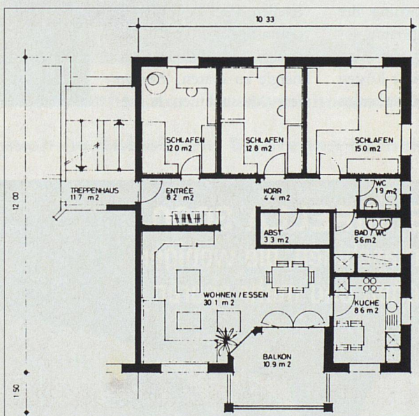
Typengrundriss B 2, 4 1/2-Zimmer-Wohnung, Bruttowohnfläche 115,5 m²; Nettowohnfläche 98,6 m²
